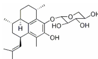
Fig. 5. Pseudopterosins A.
